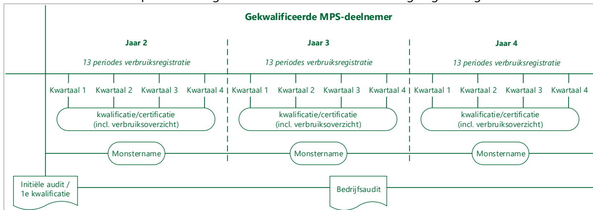
Figuur 2: Audit- en certificatieproces gecertificeerde MPS-ABC deelnemers
